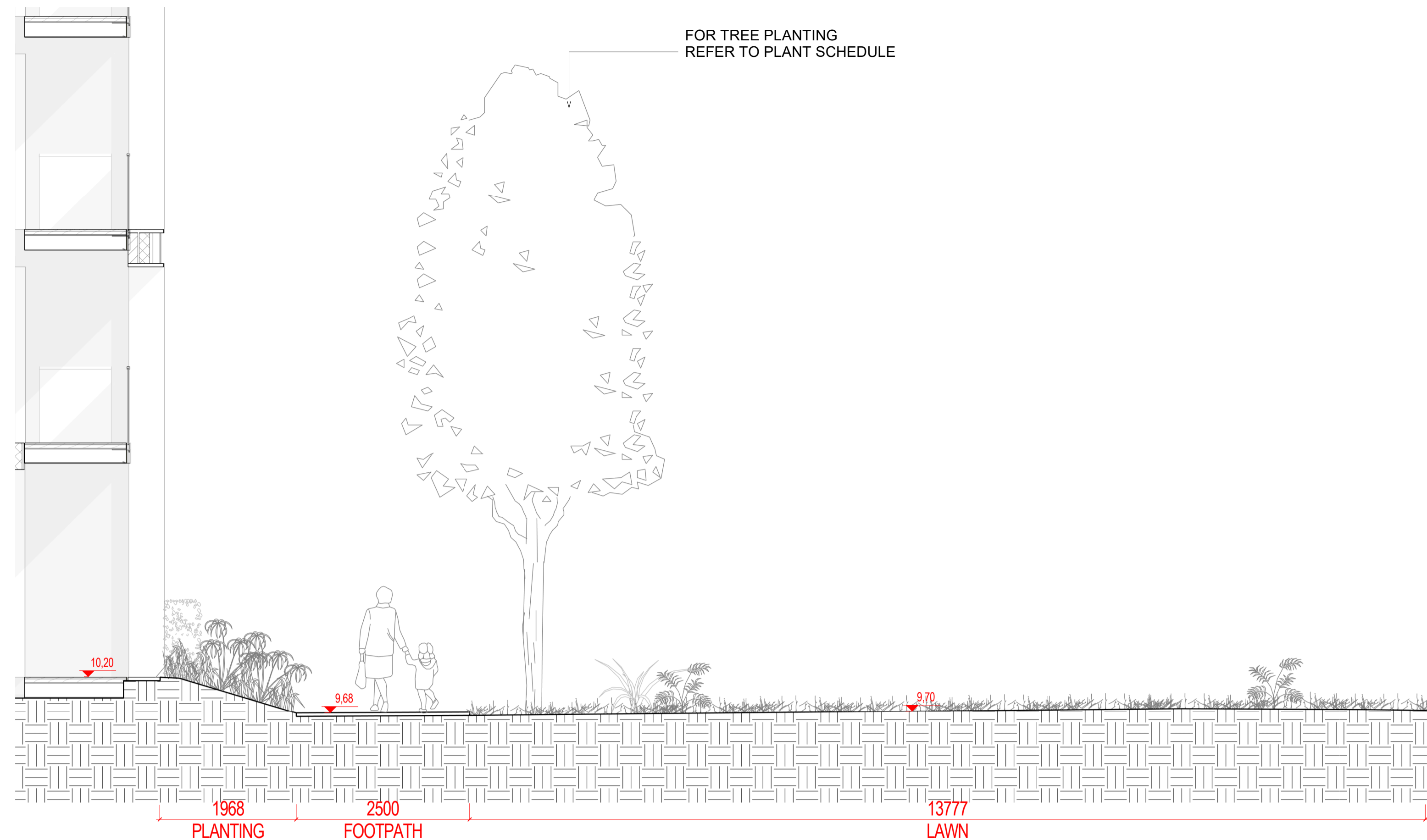
1 SECTION 29 1:50 @A1
