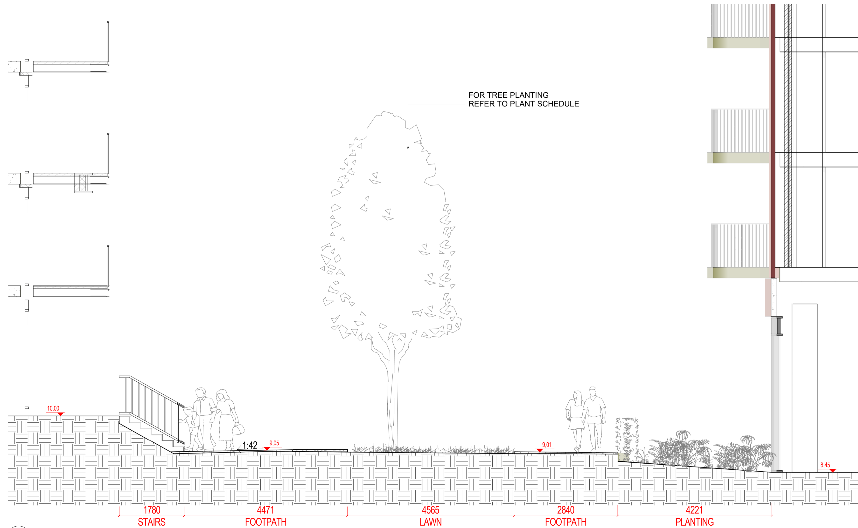
2 SECTION 30 1:50 @A1
